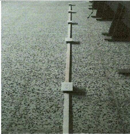
Foto 7: Mejoramiento de caja de toma corriente en centro de computo
